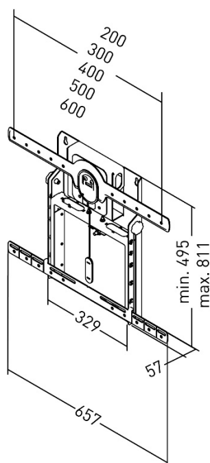
Tiroir fermé / Rack closed / Gehäuse zu
