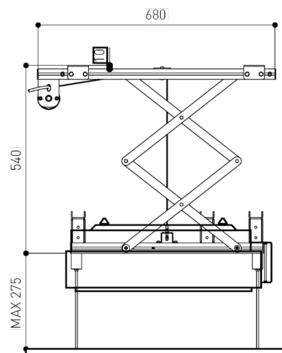
Vue latérale ouverte Side view opened
